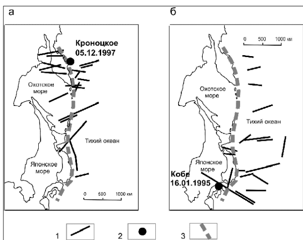
Рис. 3. Поля ЛОА в периоды, предшествующие Кроноцкому (а) и Кобе (б) землетрясениям [16]:
