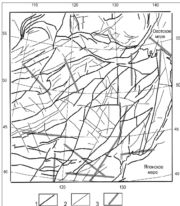
Рис. 2. Совмещение ЛОА [16] с разломами Приамурья и Северо-Восточного Китая [4, 27]:
