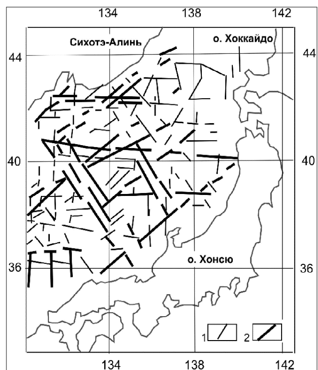
Рис. 4. Регматическая сеть разломов дна Японского моря [29]:
