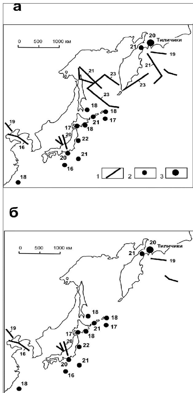
Рис. 6. Активизация Японского и Курило-Камчатского сейсмических поясов в период с 16 по 23 апреля 2006 г. На схеме: а – показаны ЛОА за весь период; б – до катастрофического землетрясения в Тиличиках 20.04.2006 [17]:
